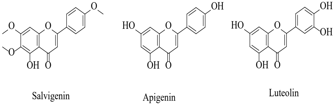
Şekil 2.3. S. palaestina 'da tespit edilen bazı flavonoitler
