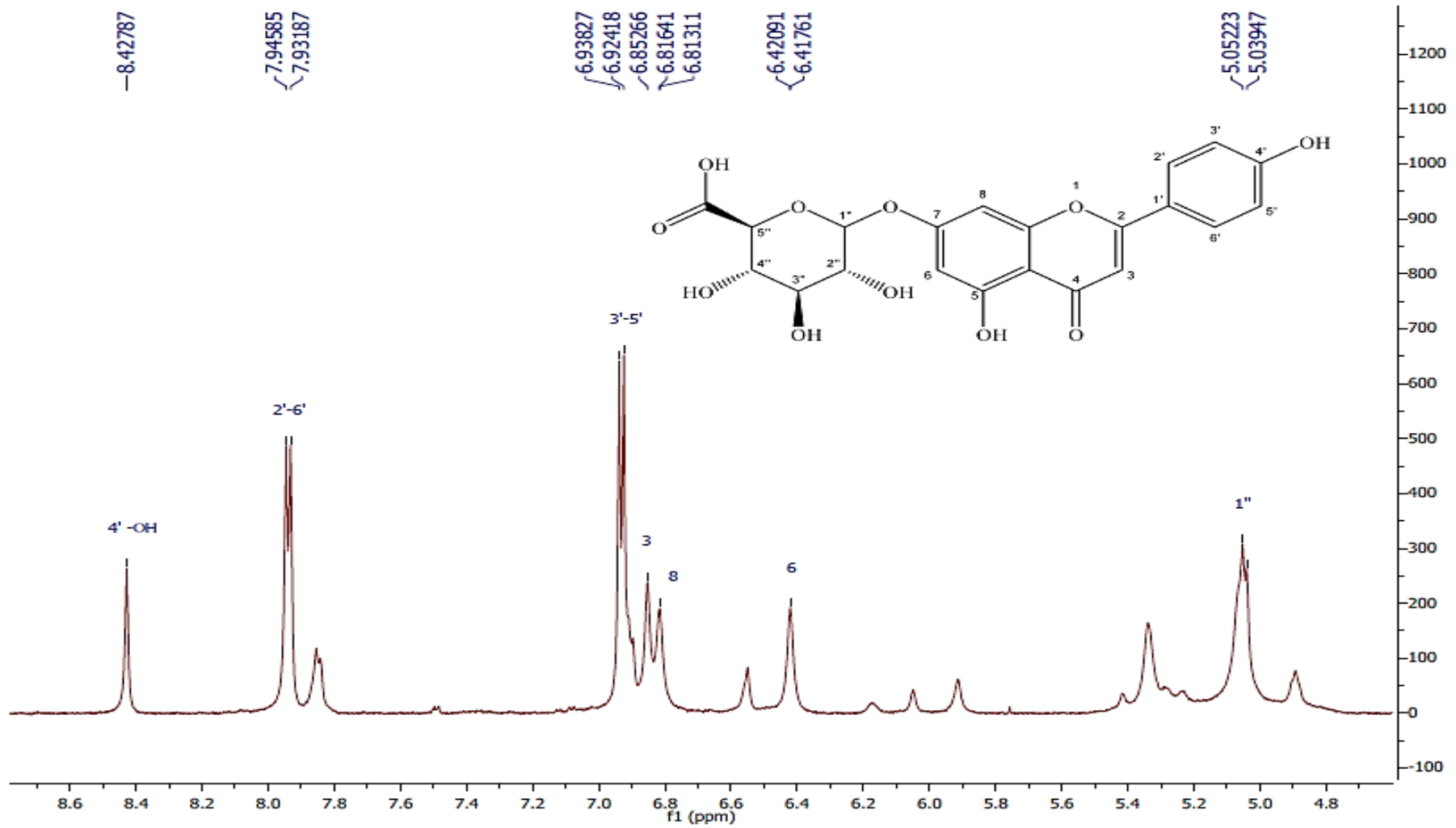
Şekil 4.26. Madde 4'e (apigenin 7-O-glukuronit) ait yakınlaştırılmış (4.8-8.6 ppm) ^1\text{H-NMR} spektrumu (DMSO- d_6 , 600 MHz)
