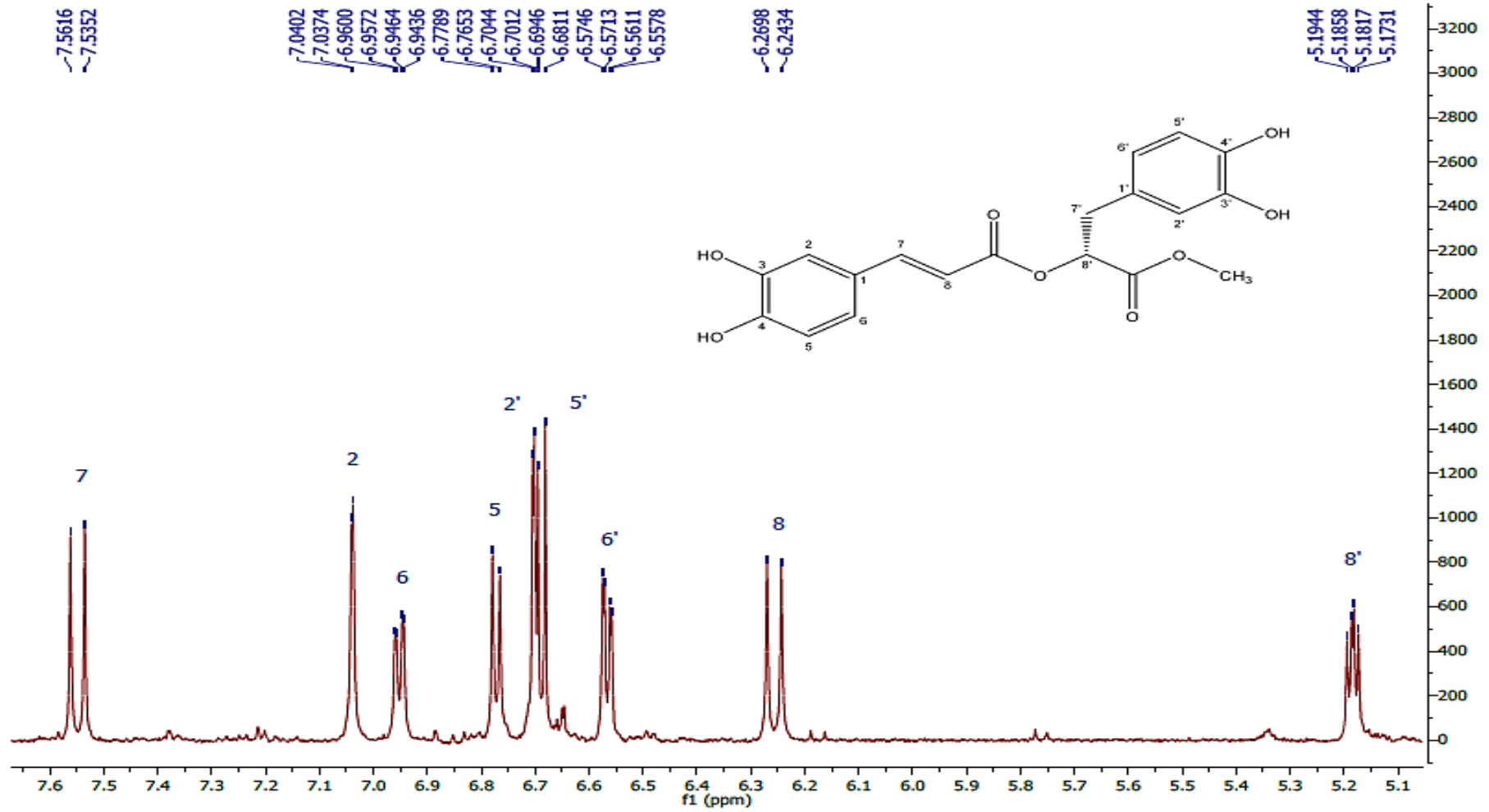
Şekil 4.12. Madde 2'ye (metil rozmarinat) ait yakınlaştırılmış (5.1-7.6 ppm) 1 H-NMR spektrumu (CD 3 OD, 600 MHz)
