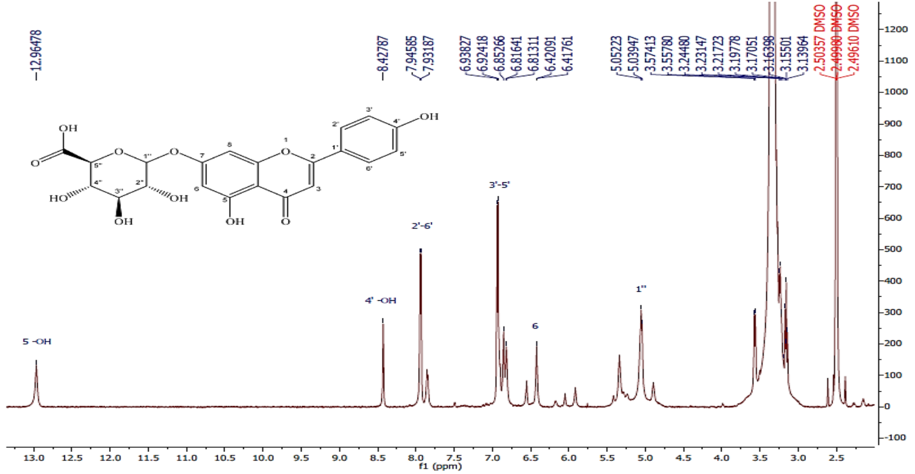
Şekil 4.25. Madde 4'e (apigenin 7-O-glukuronit) ait ^1\text{H-NMR} spektrumu (DMSO- \text{d}_6 , 600 MHz)
