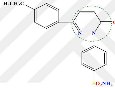
Şekil 2.31.Bileşik33'ün yapısı
