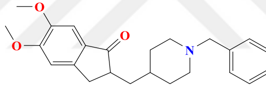
Şekil 2.9.Donepezilin yapısı
