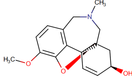
Şekil 2.10. Galantaminin yapısı
