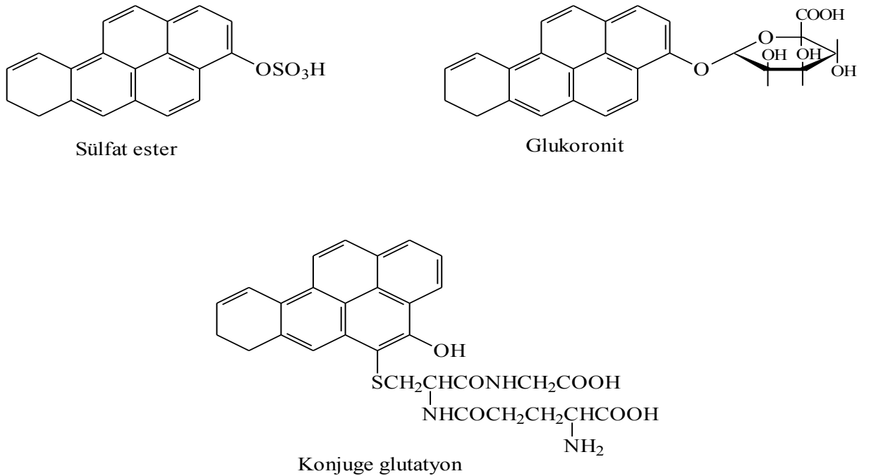
Şekil 2.2. Benzo[a]piren' in bazı konjuge biçimlerinin kimyasal yapısı (20).
