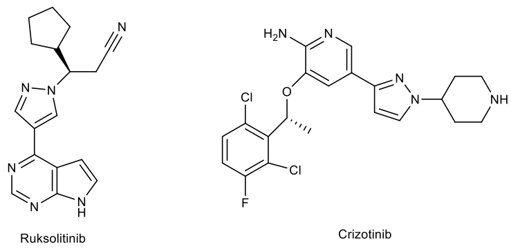
Şekil.2.3. Klinikte kullanılan pirazol yapısı içeren bazı ilaçlar
