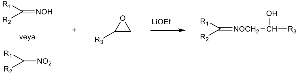
Şekil 2.39. O-Alkilasyon reaksiyonu ile oksim eter sentezi
