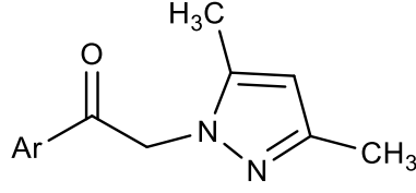
Şekil 1.2. 2-Pirazol 1-ariletanon türevi bileşiklerin ana yapısı
