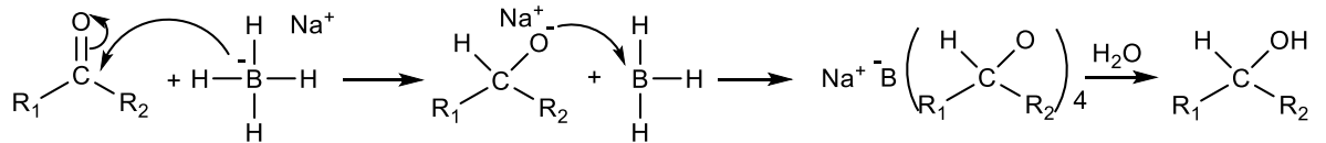
Şekil 5.5. Alkol türevlerinin sentez mekanizması
