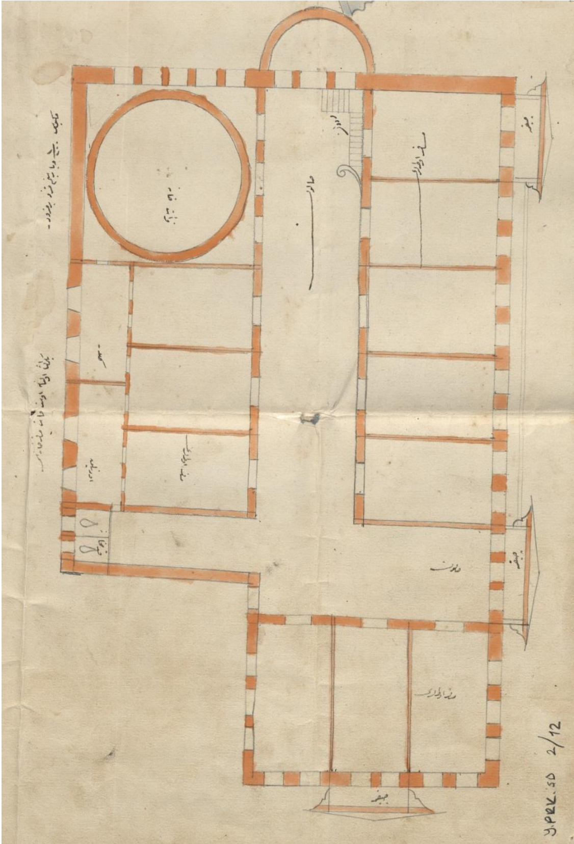
BOA., Y.PRK. ŞD., 2/12, 08 L 1312, (4 Nisan 1895). Çarşı merkezinde yeniden yapılan maârif dükkânlarının üstünde yapılması düşünülen misafirhanenin kat planı.
