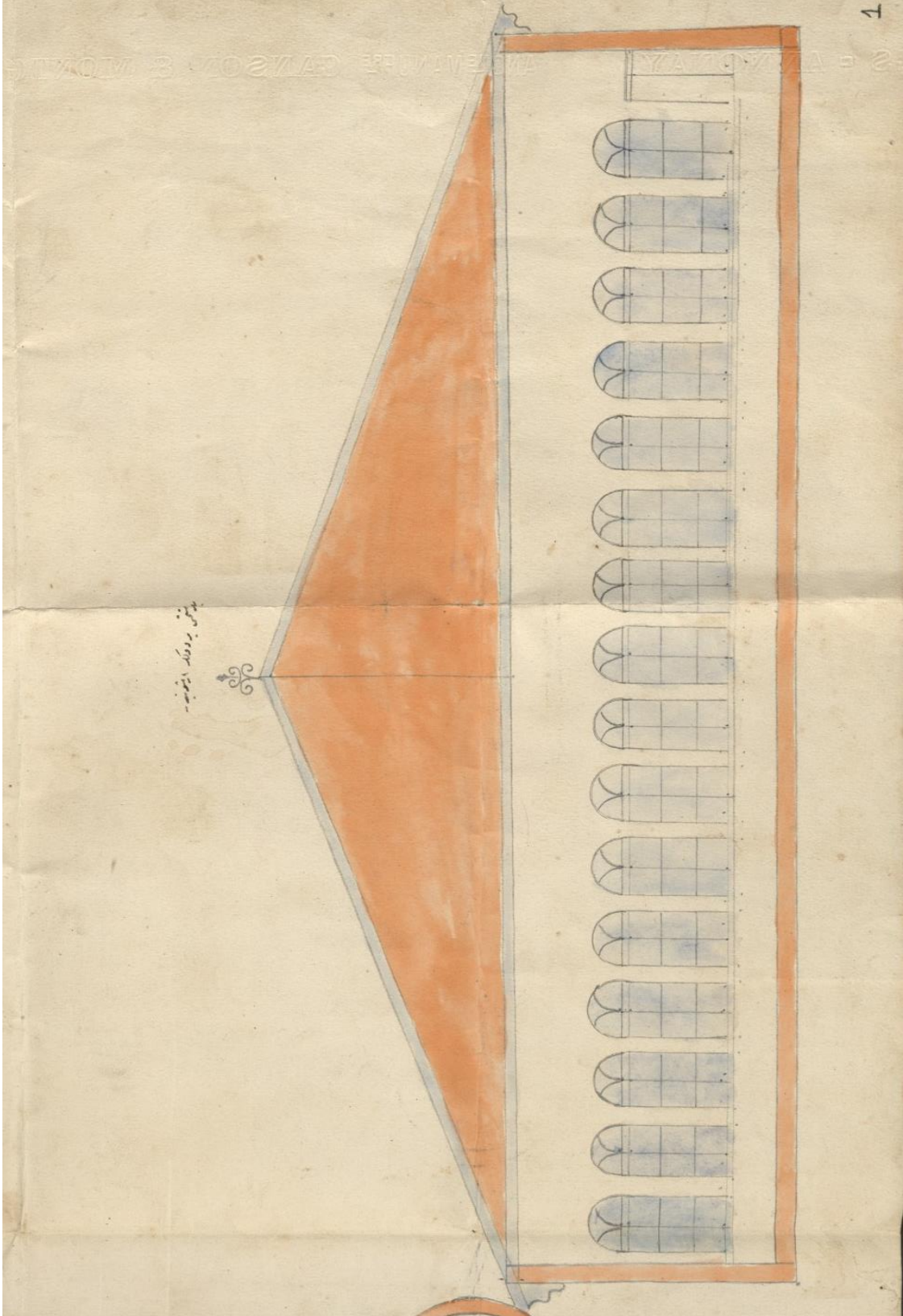
BOA., Y.PRK. ŞD., 2/12, 08 L 1312, (4 Nisan 1895). Çarşı merkezinde yeniden yapılan maârif dükkânlarının üstünde yapılması düşünülen misafirhanenin dıştan görünüşü.
