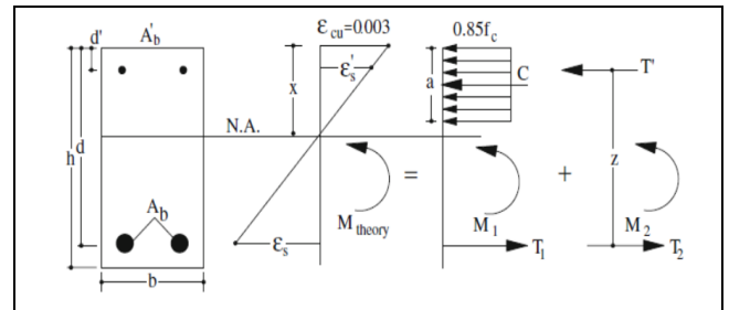
Şekil 6. Betonarme kirişlerde gerilme-şekil değiştirme dağılımı
