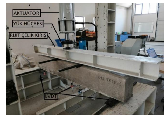
Şekil 5. Kiriş numunesi test düzeneği.
